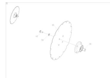
ЕТВ-6000000183, Диск
