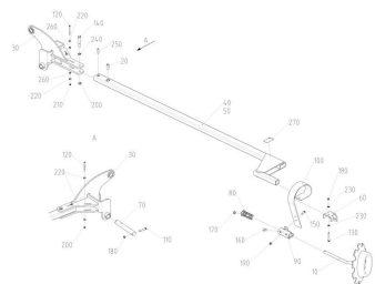
ЕТВ-6000000392, Стрела
