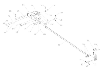
ЕТВ-6000000391, Тяга
