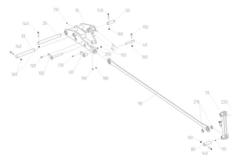
ЕТВ-6000000391, Тяга
